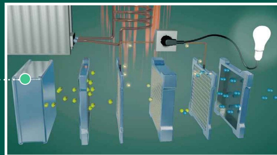
Aus Erdgas und Sauerstoff entstehen Strom und Wärme.
